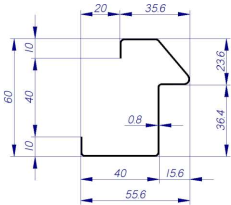
Przekrój ościeznicy CS4
