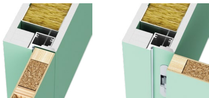
Bezprzylgowe standard (otwierane na zewnątrz) – drzwi prawe
