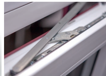
Zasuwnica komfort
