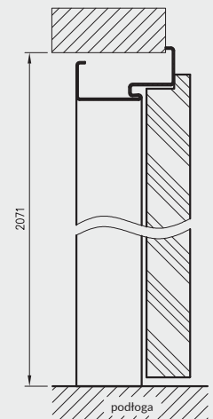
Przekrój pionowy alternatywny sposób montażu
