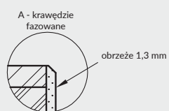
Przekrój ramiaka skrzydła bezprzylgowego
