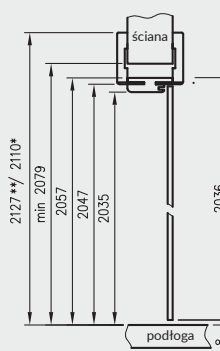
Przekrój pionowy drzwi szklanych z ORC
