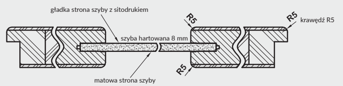
Przekrój poziomy drzwi VETRO B5, B10-B11
