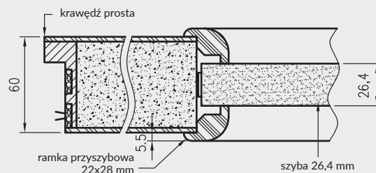
Skrzydło drzwiowe przeciwpożarowe Olimp EI60
