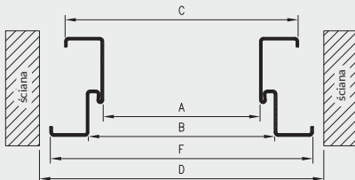
Przekrój poprzeczny
